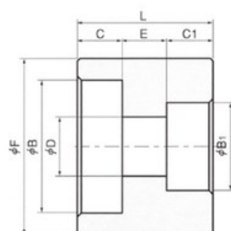
同心
