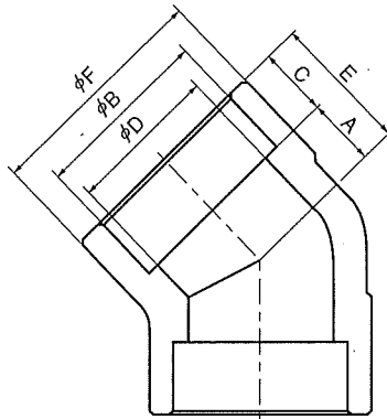
45°エルボ
